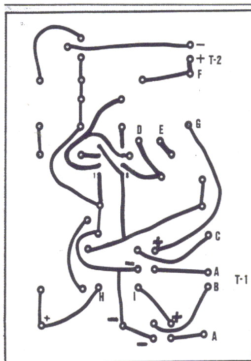
PLACA DE CIRCUITO IMPRESSO VISTA DE BAIXO
